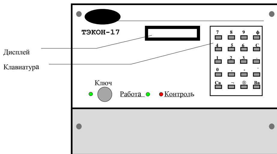
Рисунок 2.1 – ТЭКОН-17 с клавиатурой и цифробуквенным ЖКИ индикатором
