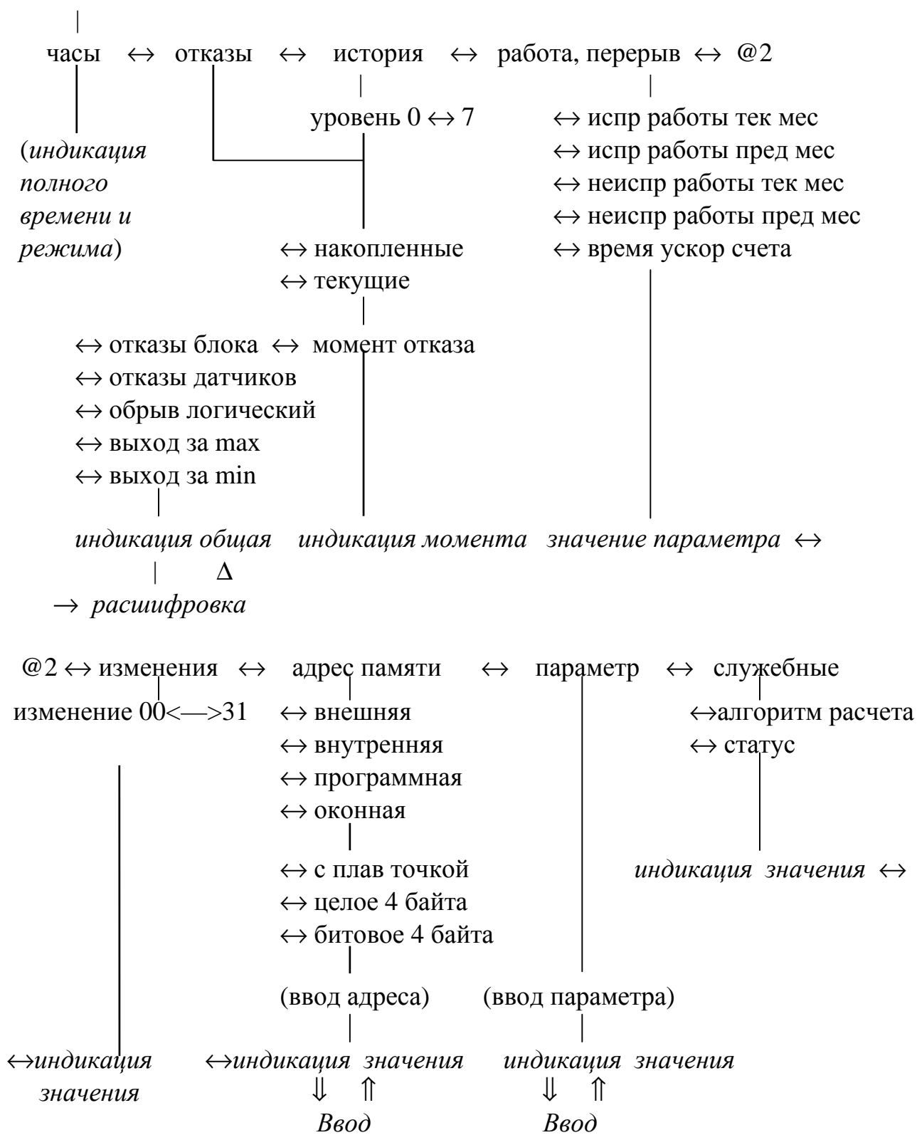
Рисунок 4.6 – Раздел меню КОНТРОЛЬ
