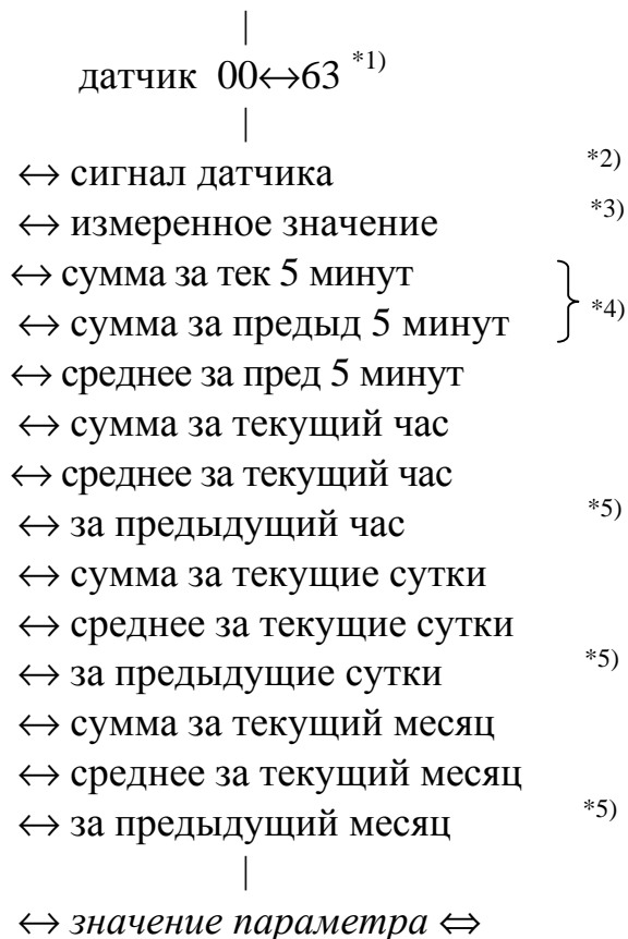
Рисунок 4.3 - Раздел меню ИЗМЕРЕНИЕ
